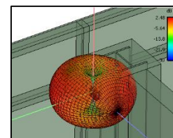
Точка доступа (2.45 GHz, 23 dBm Conducted Power)
