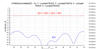
Согласование и изоляция широкополосного делителя
