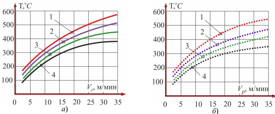
Рисунок 3. Влияние скорости резания и различных составов СОТС на температуру резания:
