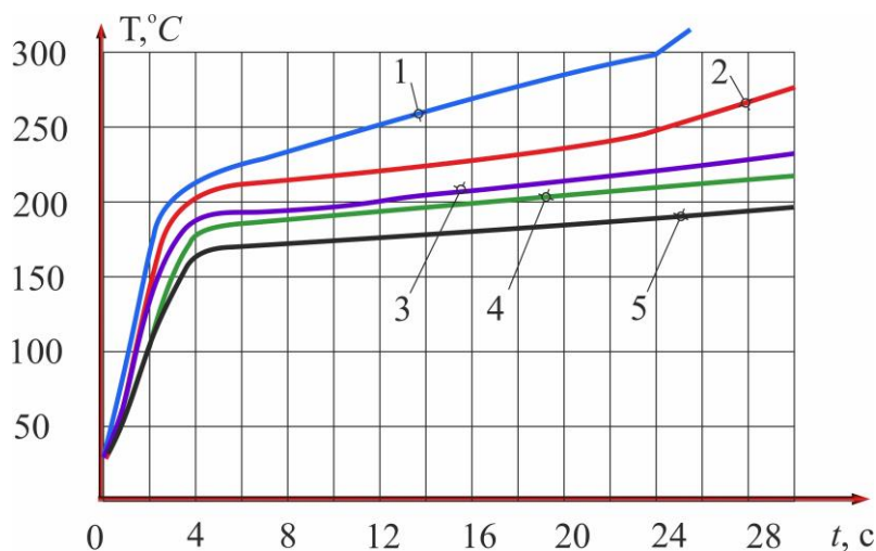
Рисунок 5. Зависимость температуры режущих кромок сверла от времени при подаче различных СОТС: Режимы резания: V = 11 м/мин; S = 0,076 мм/об. Расход СОТС 0,5 л/мин. Режущий инструмент Р6М5. 1 – «сухое резание»; 2 – минеральное масло И-20А; 3 – минеральное масло И-20А с НГМП; 4 – подсолнечное масло; 5 – подсолнечное масло с НГМП.
