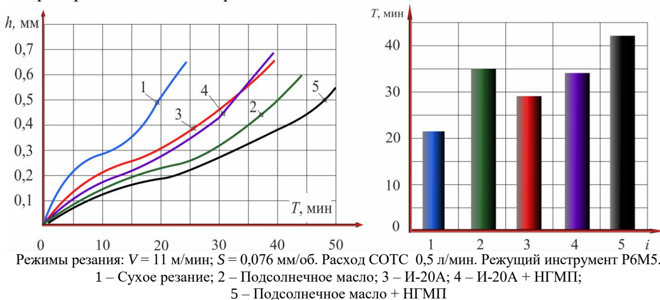
Рисунок 8. Влияние различных составов СОТС на износ задней поверхности и стойкость сверла из быстрорежущей стали Р6М5 при обработке стали 12Х18Н10Т.
