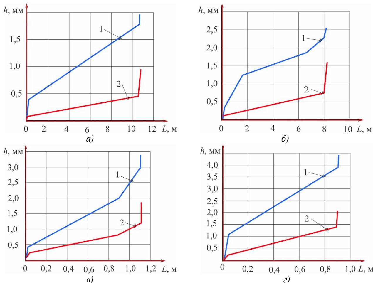
Рисунок 7. Зависимость среднего износа по задней поверхности сверла и износа у уголков от суммарной глубины отверстий при сверлении: 1 – износ у уголков; 2 – средний износ по задней поверхности; а) V = 11 м/мин и S = 0,076 мм/об.; б) V = 21 м/мин и S = 0,076 мм/об.; в) V = 31 м/мин и S = 0,076 мм/об.; г) V = 41 м/мин и S = 0,076 мм/об.
