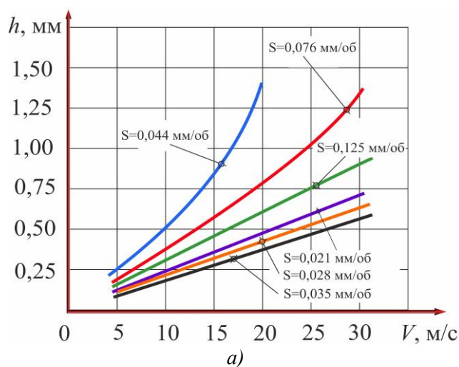
Рисунок 6. Зависимости предельного износа спиральных сверл диаметром 22 мм от режимов обработки стали 12Х18Н10Т: а) подача СОТС по каналам сверла; б) подача СОТС поливом.
