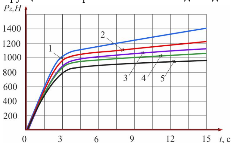
Рисунок 4. Зависимость тангенциальной силы резания P_z при сверлении стали 12Х18Н10Т в условиях подачи различных СОТС:
