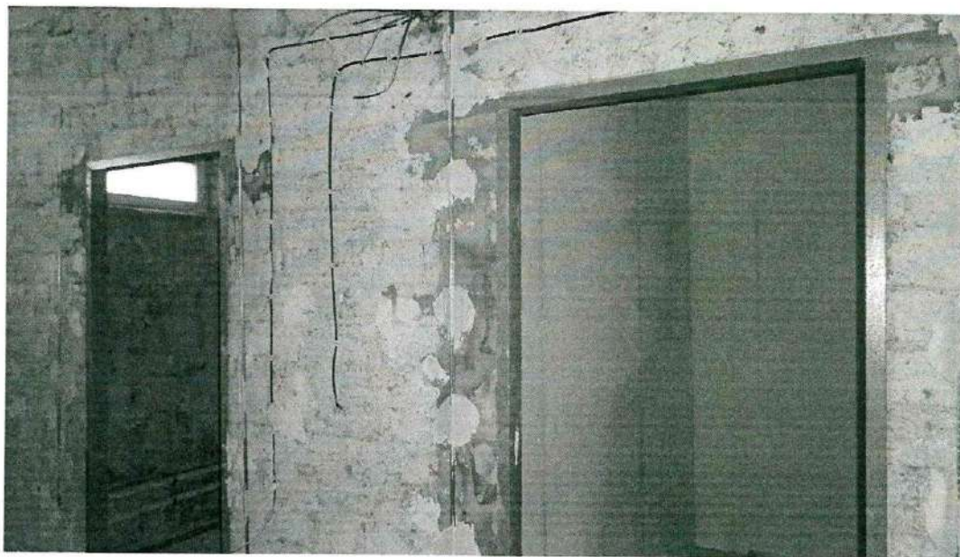
Работы по усилению дверных проемов.
