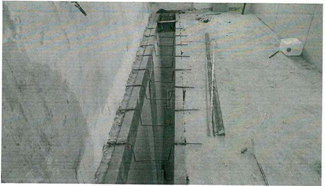
Работы по устройству вентканалов.
