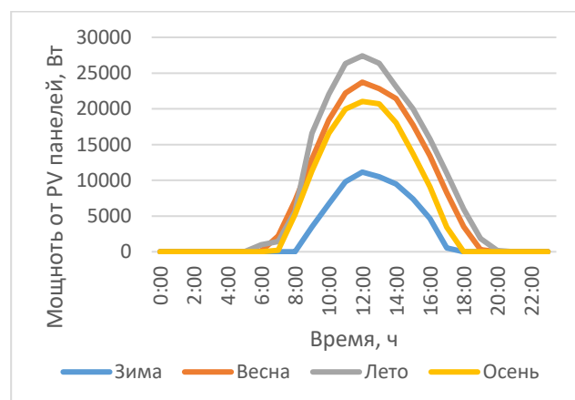
Рис. 6 Мощность от солнечных батарей за сутки
