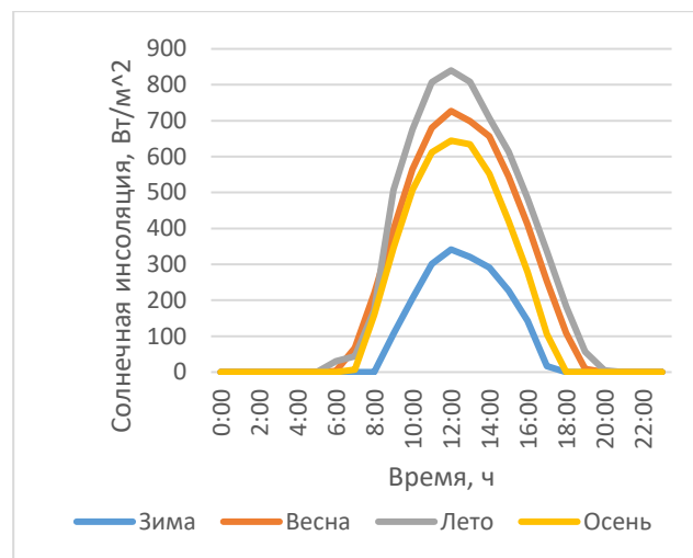
Рис. 5 Солнечная инсоляция за сутки
