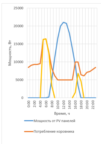
Рис. 7. График потребления и выработки электроэнергии (весенний период)
