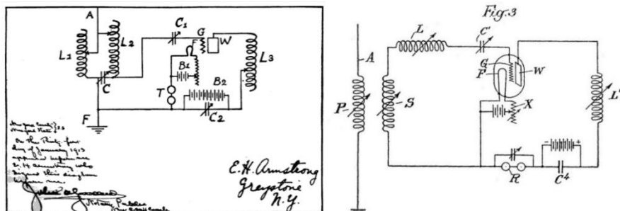
Рис. 5. Регенеративная схема Армстронга (слева), нотариально заверенная 31 января 1913 г. [16]. Одна из принципиальных схем регенеративного приемника (справа) из патента Э. Армстронга US1113149A [15].
