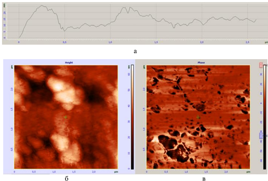
Рис. 1. а — профиль сечения фольги, иллюстрирующий характер неровностей в средней части выбранной области; б — изображение участка фольги, полученное в АСМ, иллюстрирующий характер неровностей поверхности фольги размером 2,5 \times 2,5 мкм; в — изображение того же участка фольги в режиме фазового контраста АСМ.
