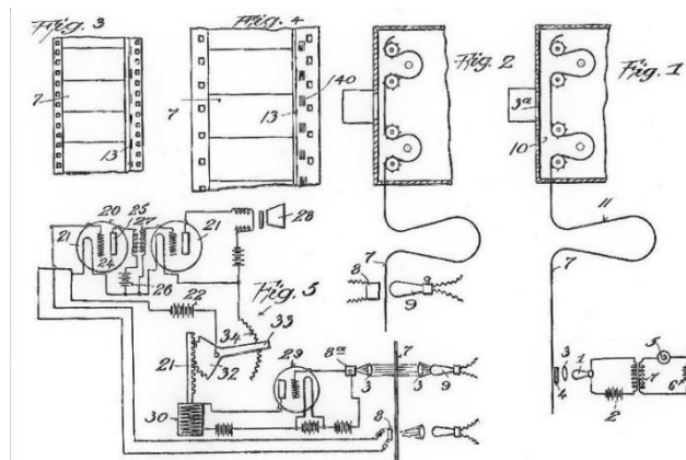
Рис. 11. Первый из множества патентов Ли де Фореста на систему Sound-on-film . Рисунок из патента US1446246A с приоритетом от 18 сентября 1919 г. [23].
