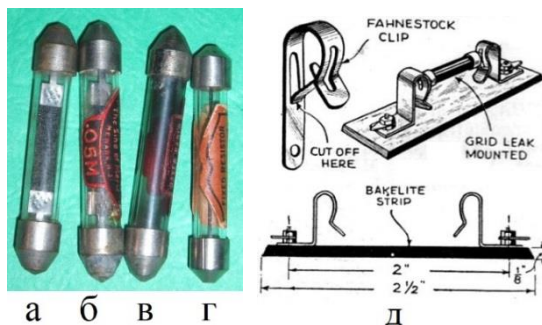
Рис. 7. Типичные утечки сетки: а, б — с пропитанными бумажными элементами, в — с внутренним покрытием, г — с покрытием внутренней поверхности стеклянной трубки и д — устройство монтажа гридлика.
