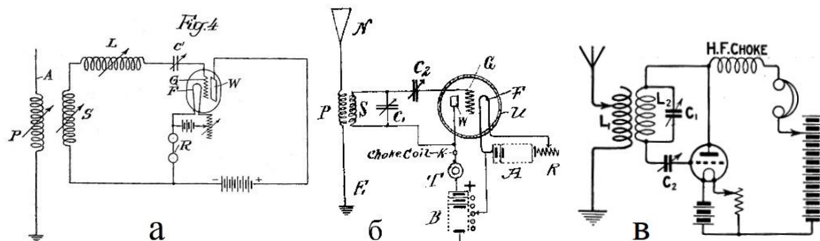
Рис. 3. Схема приемника Поля Уоллеса (а) из патента US1113149A Эдвина Армстронга [12]. Схема регенеративного приемника Ultra-Audion (б) из патента US1170881A Ли де Фореста [13]. Современное условно-графическое исполнение схемы регенеративного приемника Ultra-Audion (в) Ли де Фореста.
