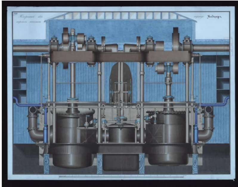
Рис. 1. «Поперечный вид паровым машинам» пароходофрегата Владимир. РГАВМФ. Ф. 327. Оп. 1. Ед.хр. 1838.
