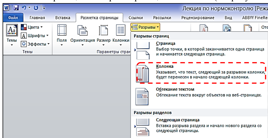
Рисунок 7 – Инструменты MicrosoftWord
