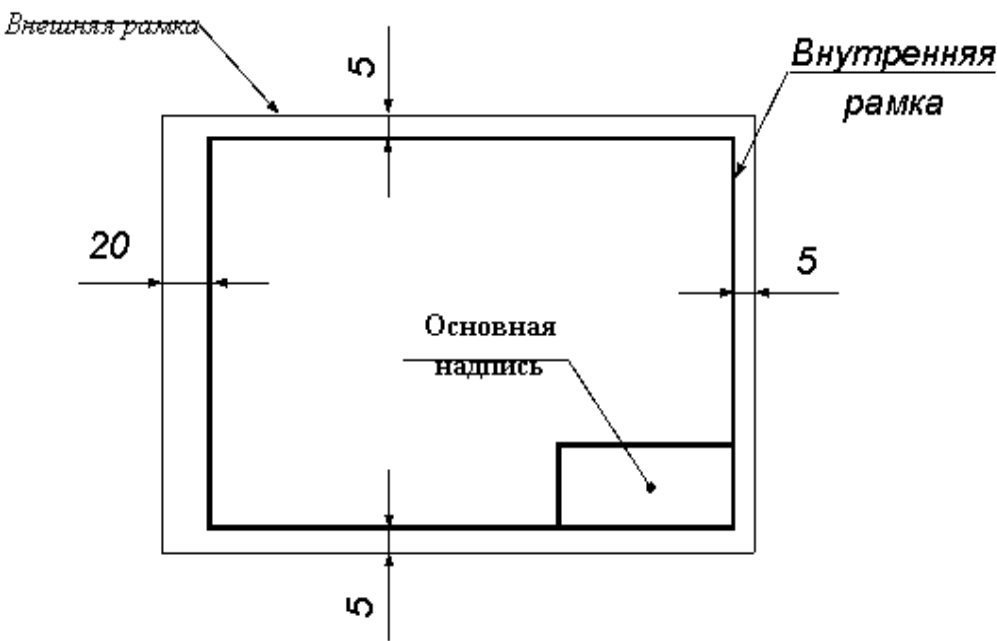
Рисунок Д.1 – Параметры рамки чертежа
