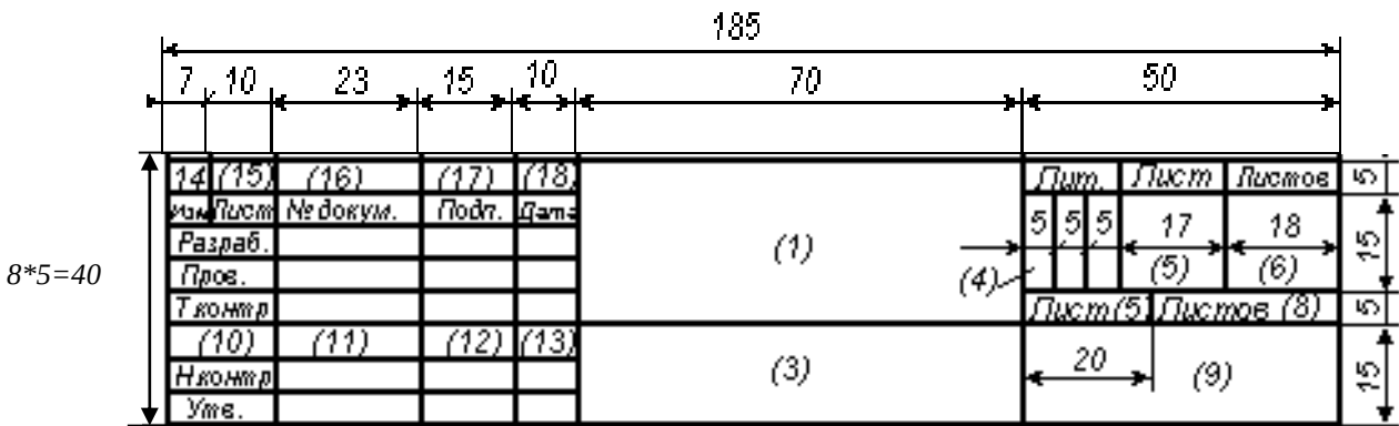
Рисунок Д.2 – Параметры основной надписи чертежа
