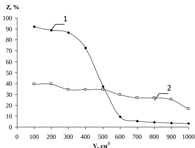
Рисунок 3.6 – Зависимость степени очистки воды от хлоридов (1) и степени умягчения (2) от пропущенного через анионит АВ-17-8 в OH - –форме
