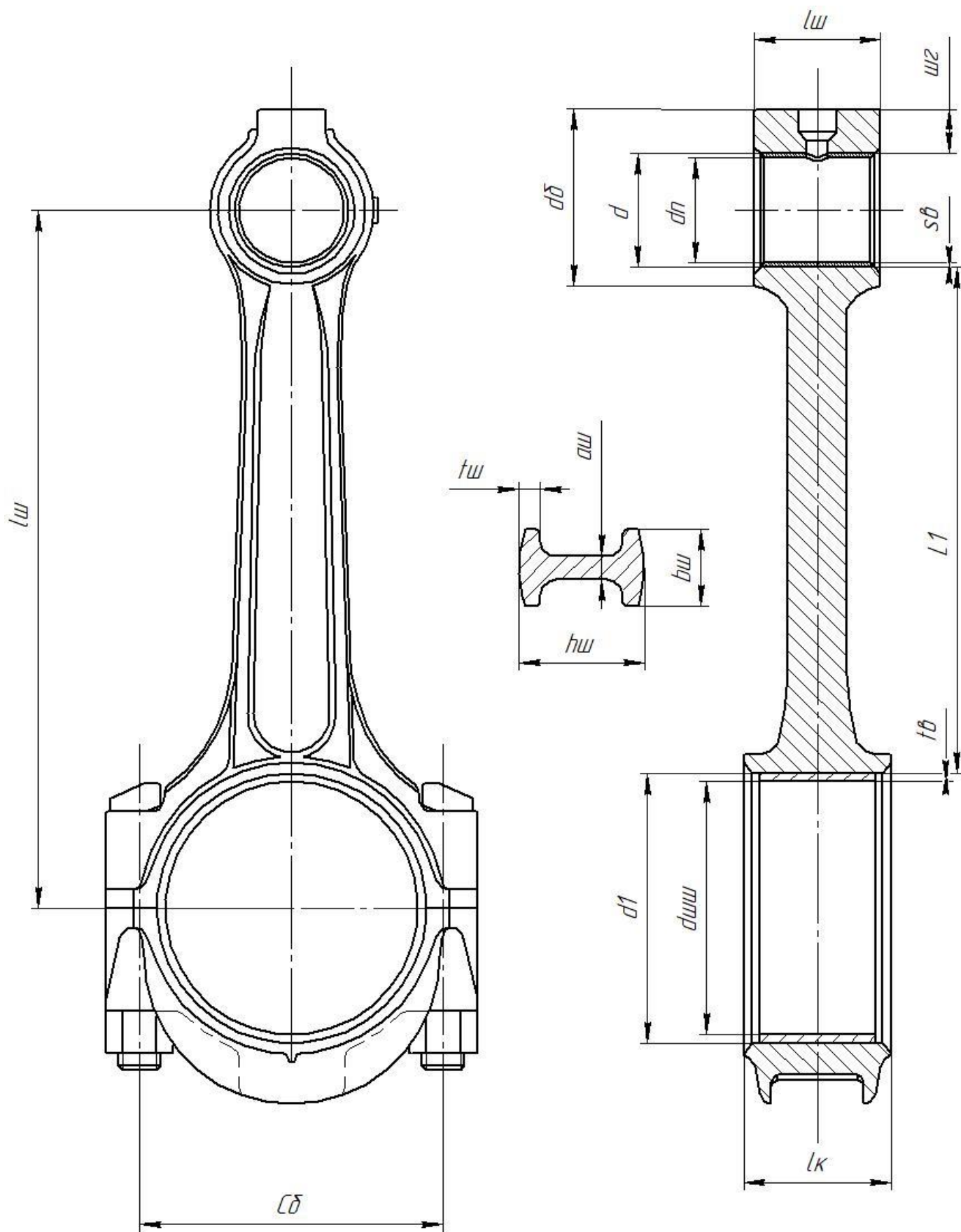
Рисунок 22- Эскиз детали шатун
