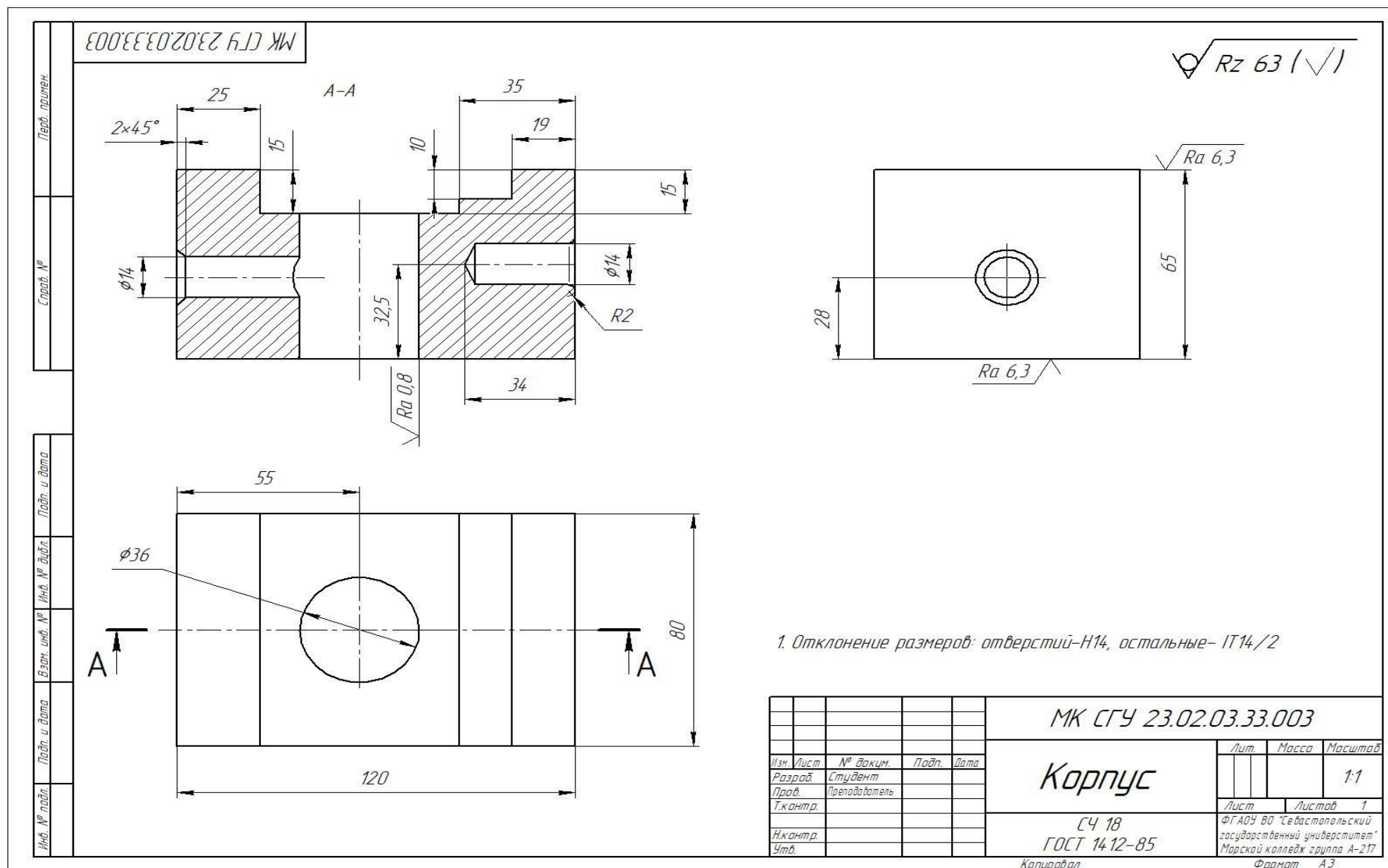
Рисунок 8- Пример выполненного чертежа детали корпус
