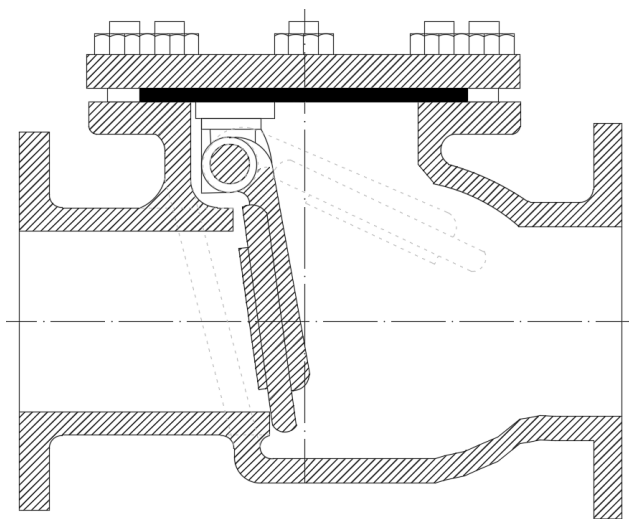
Рис. 11. Захлопка
