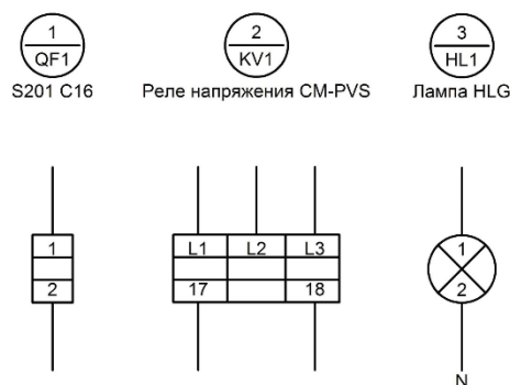
Рисунок 4- Вид элементов для монтажной схемы Э4
