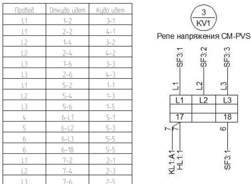
Рисунок 5- Таблица соединений и элемент на монтажной схеме с подключением
