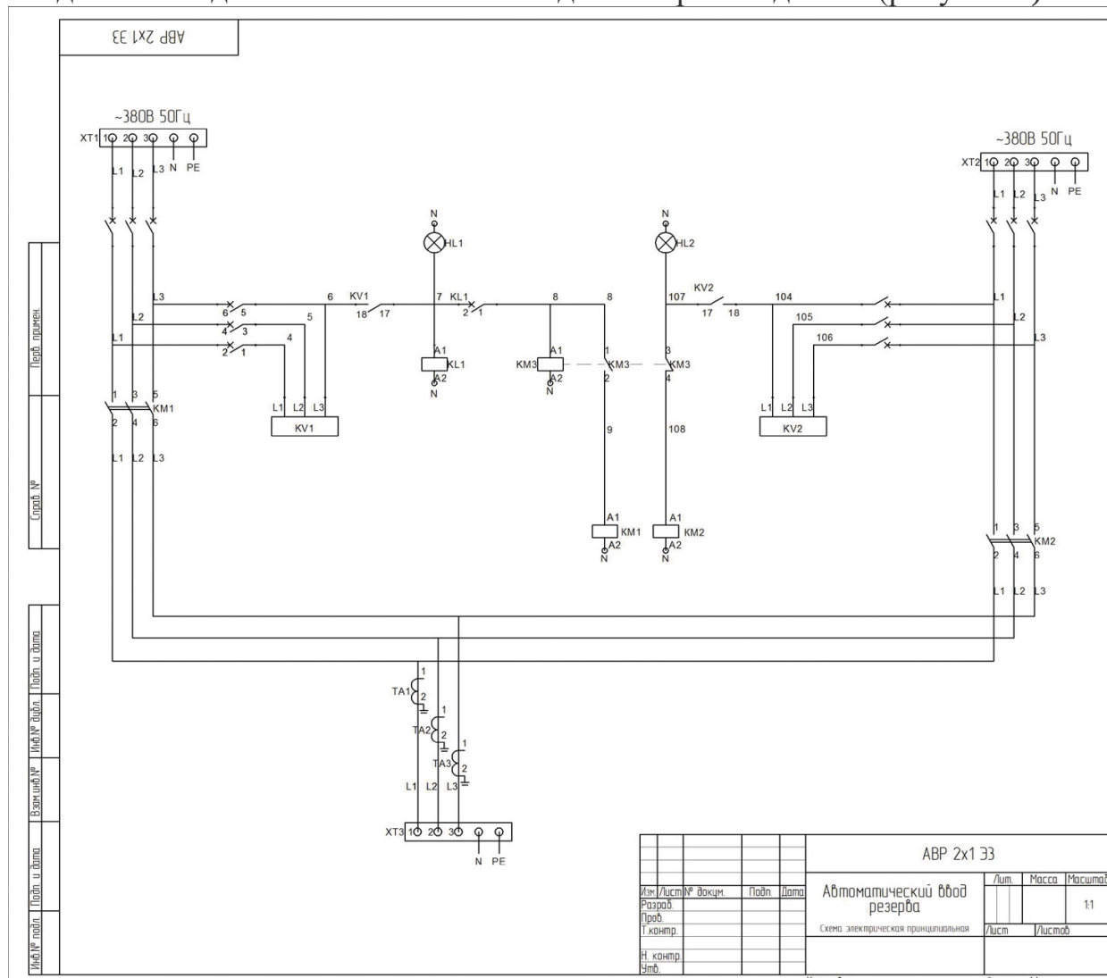
Рисунок 1 -Принципиальная электрическая схема
