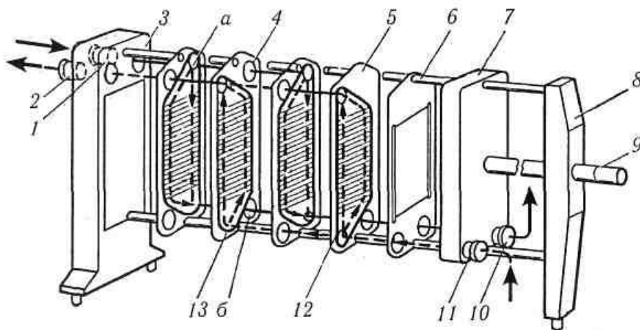
Рис. 7. Пластинчатый теплообменник
