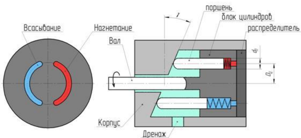
Рис. 5. Аксиально-поршневой насос с наклонным диском
