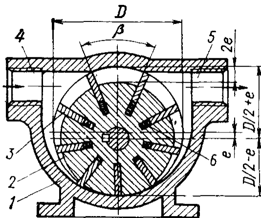
Рис. 1. Пластинчатый насос однократного действия
