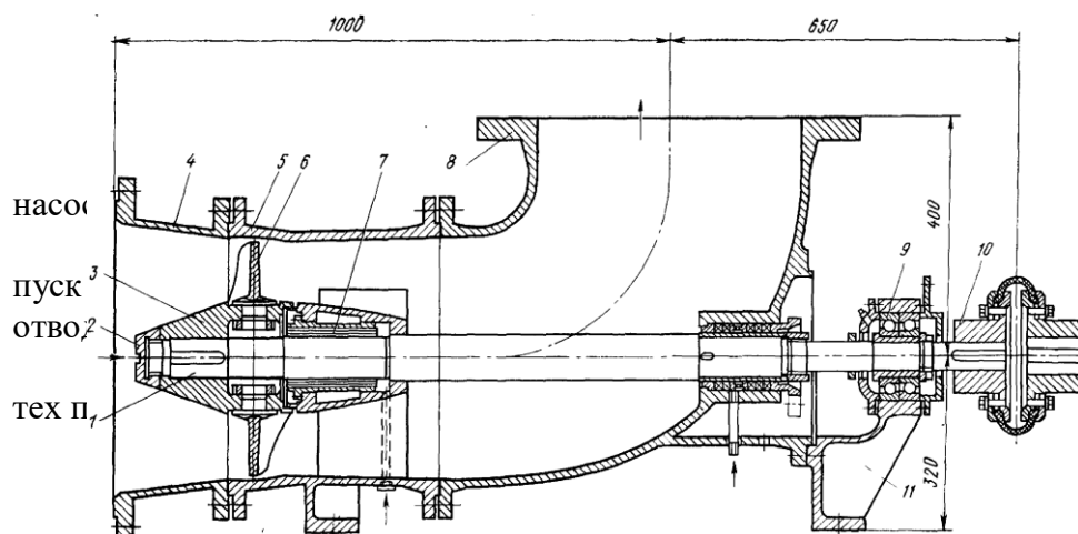
Рис. 3. Горизонтальный осевой насос
