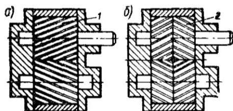
Рис.3. Схемы насосов с косозубыми и шевронными шестернями
