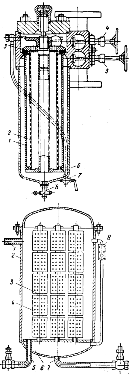
Рис. 15. Емкостный фильтр
