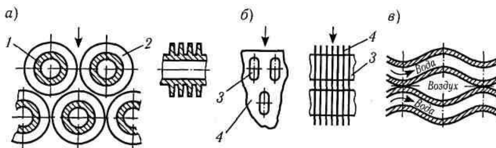
Рис. 4. Теплообменные поверхности воздухоохлаждателей дизелей
