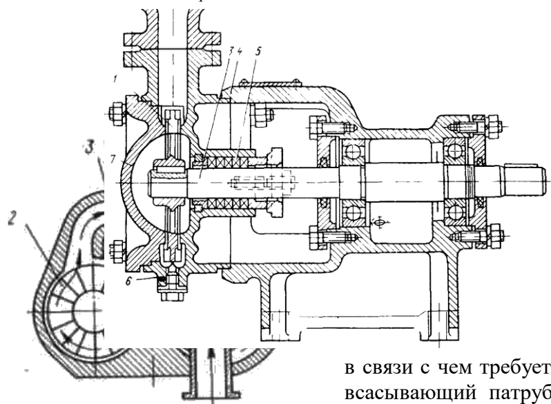
Рис. 6. Схема центробежно-вихревого насоса
