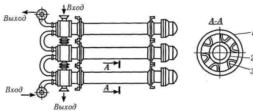
Рис. 6. Секционный подогреватель топлива
