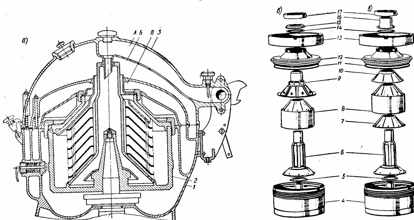
Рис.4. Барабан несамоочищающегося сепаратора типа MB1500/1700C «Де Лаваль»
