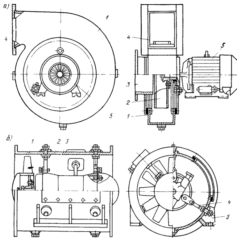
Рис. 1. Схемы электровентиляторов
