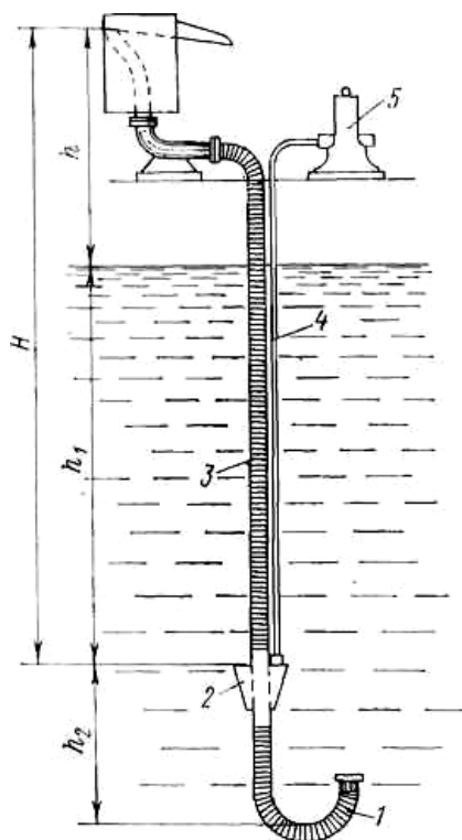
Рис. 3. Схема эрлифта
