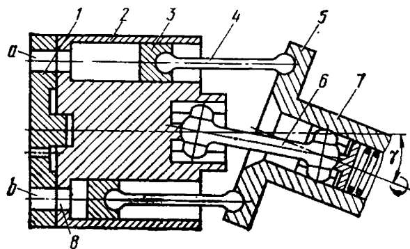
Рис. 6. Схема аксиально-поршневого насоса с наклонным диском
