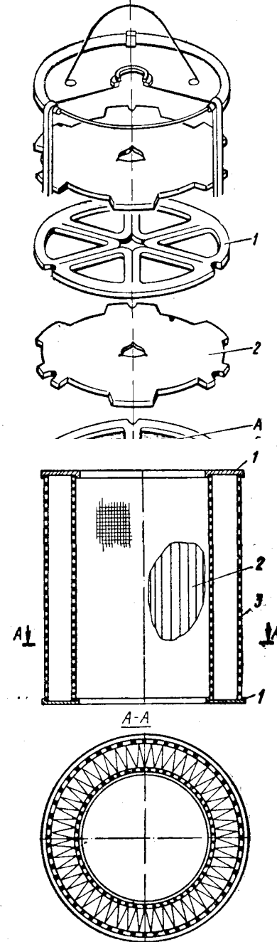
Рис. 9. Полнопроточный бумажный фильтрующий элемент: 1 – крышка; 2 – бумажный фильтрующий элемент; 3 – сетчатый цилиндр
