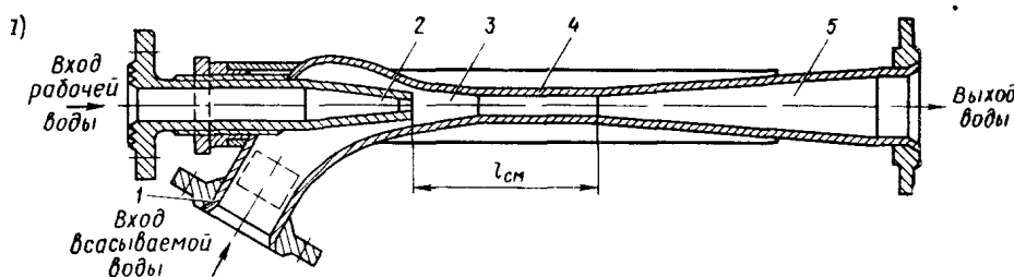
Рис.1. Водоструйный эжектор
