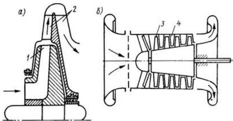
Рис. 5. Принципиальные схемы лопастных компрессоров: а — центробежного; б — осевого 1, 3 — лопастное колесо; 2 — канал; 4 — направляющий аппарат
