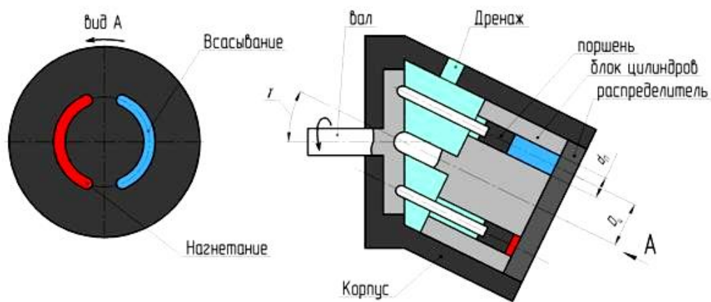
Рис.4. Аксиально-поршневой насос с наклонным цилиндрическим блоком
