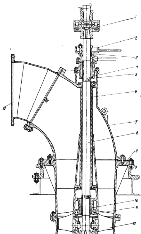
Рис. 2. Вертикальный осевой насос
