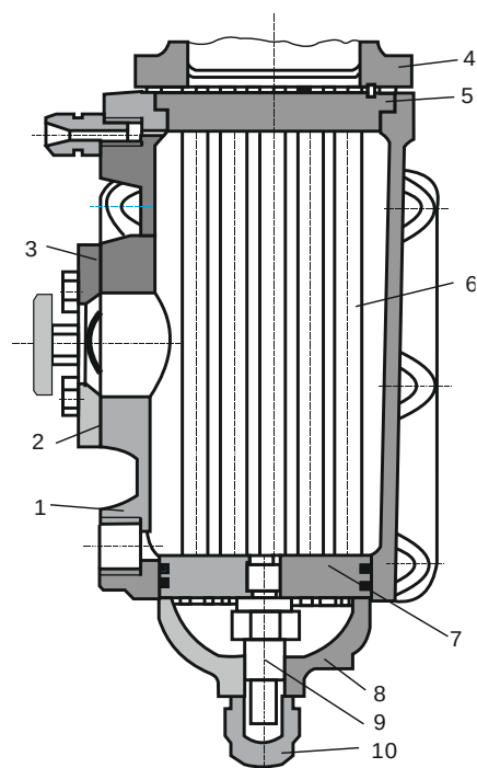
Рис. 5. Холодильник 1 ступени: 1 – корпус; 2 – крышка; 3 – мембрана; 4 – водомаслоотделитель; 5, 7 – трубные доски; 6 – трубки; 8 – крышка; 9 – шпилька; 10 – гайка глухая.
