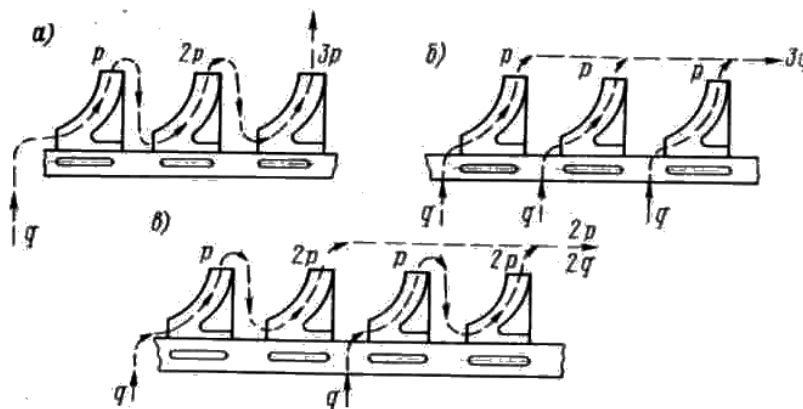
Рис. 2 Схемы соединения колес центробежных насосов: а – последовательное; б – параллельное; в – смешанное
