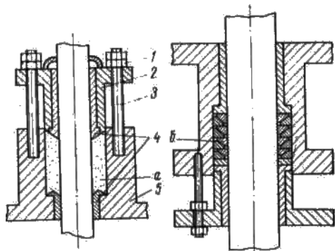
Рис. 5. Уплотнения (сальники) поршневых насосов
