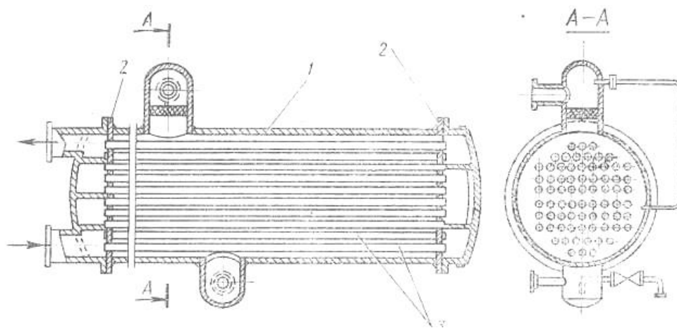
Рис. 4. Устройство кожухотрубного испарителя:
