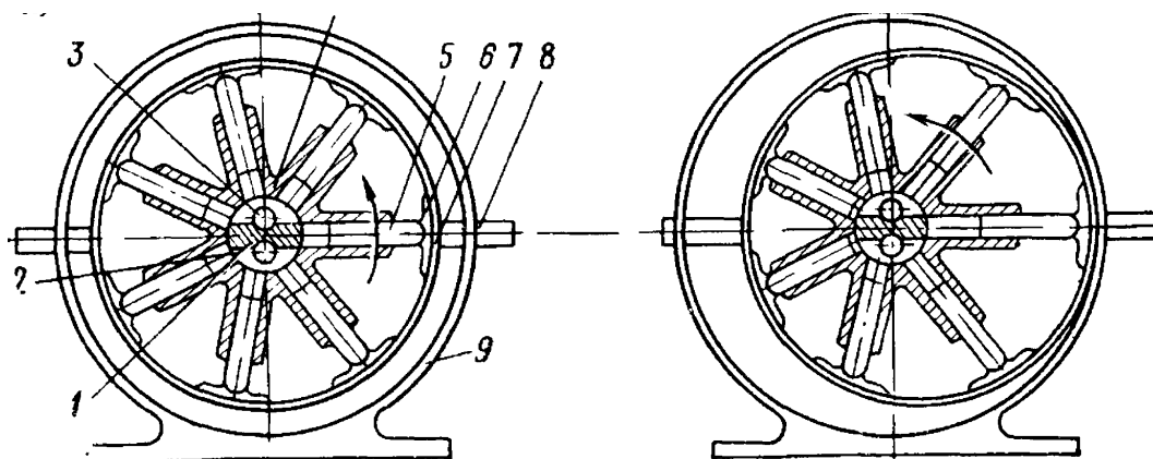
Рис. 3. Схема радиально-поршневого насоса
