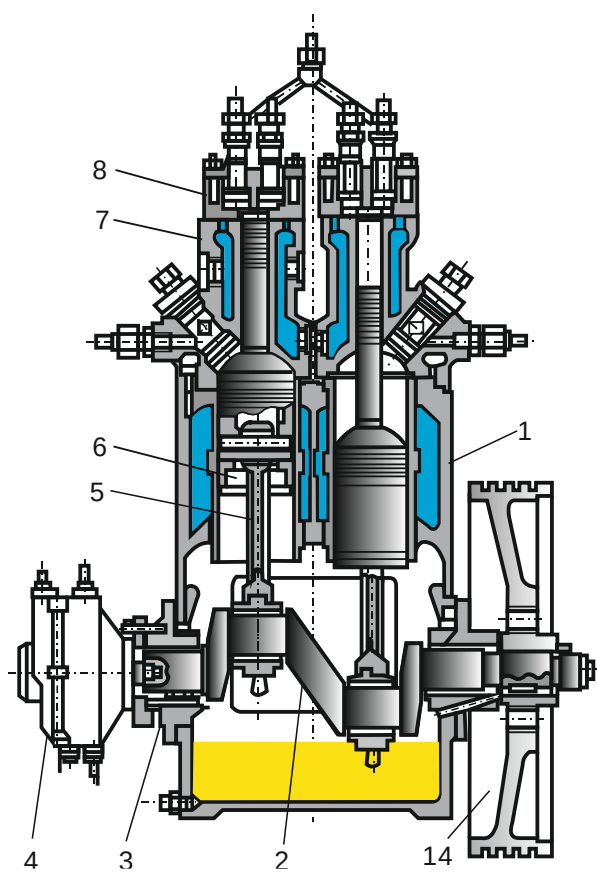
Рис. 2. Продольный разрез компрессора: 1 – станина; 2 – коленчатый вал; 3 – коренной подшипник; 4 – водяной насос; 5 – шатун; 6 – поршень; 7 – цилиндр высокого давления; 8 – крышка цилиндра; 9 – всасывающий клапан 1 ступени; 10 – клапан 2 ступени; 11 – водомаслоотделитель; 12 – холодильник 2 ступени; 13 – черпак; 14 – шкив-маховик.
