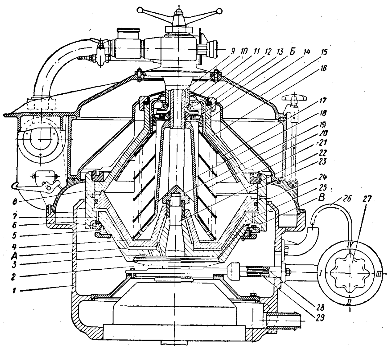
Рис. 5. Барабан самоочищающегося сепаратора МАРХ207-00S «Де Лаваль»
