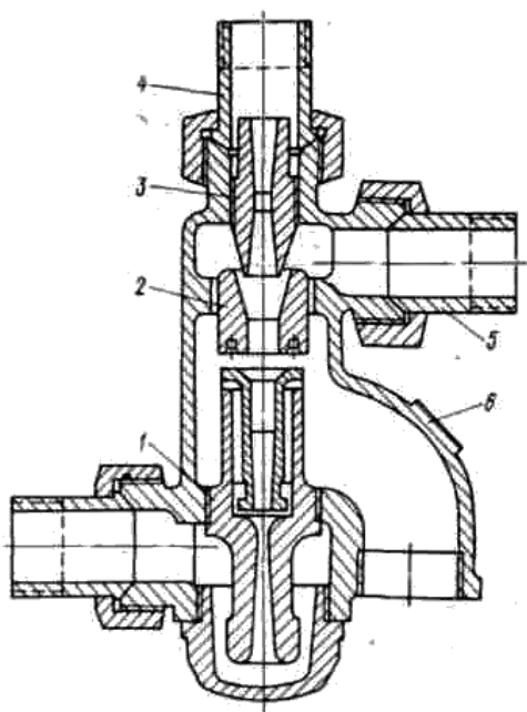
Рис. 2. Самовсасывающий инжектор
