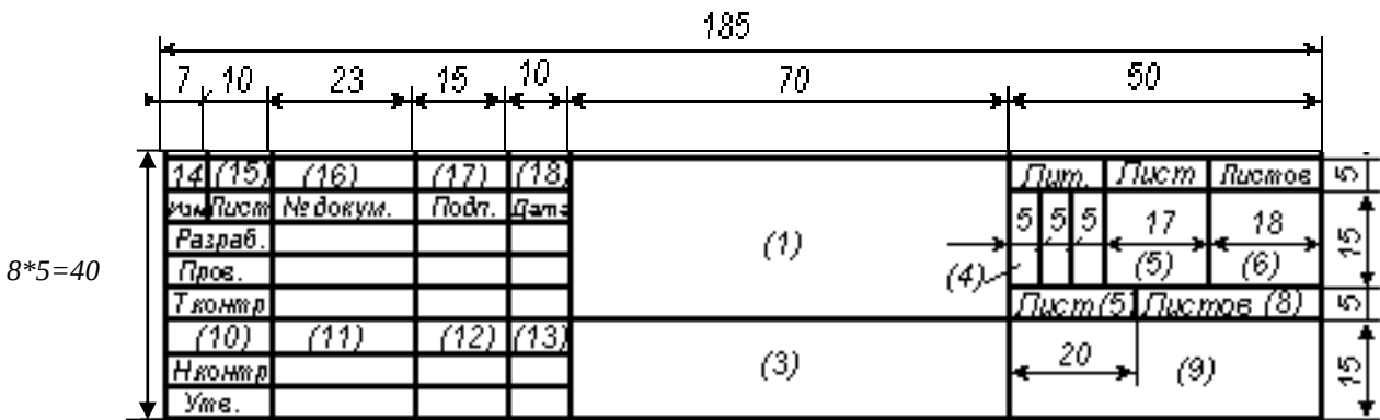
Рисунок Ж.2 – Параметры основной надписи чертежа
