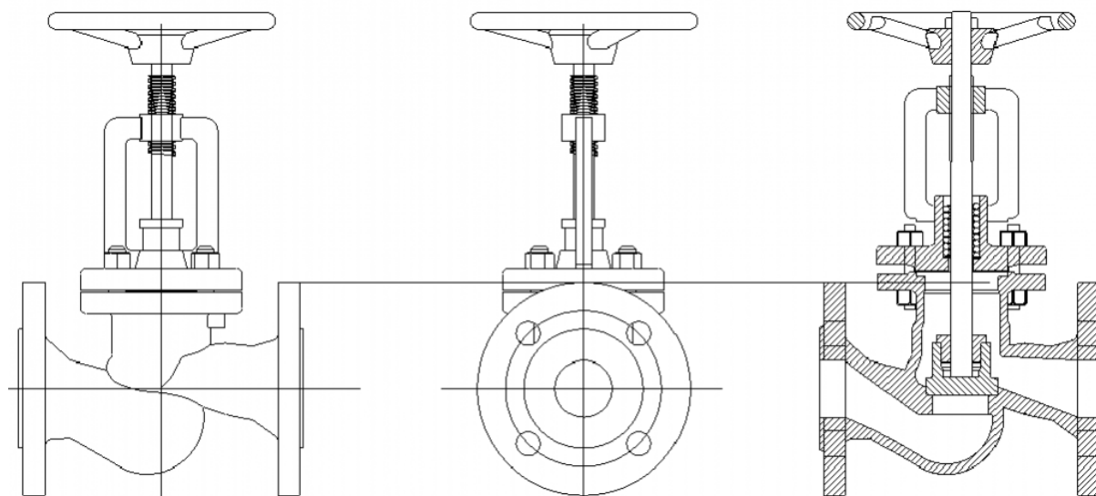
Рис. 15. Запорный клапан
