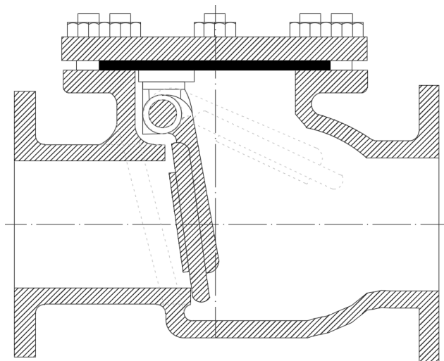
Рис. 11. Захлопка
