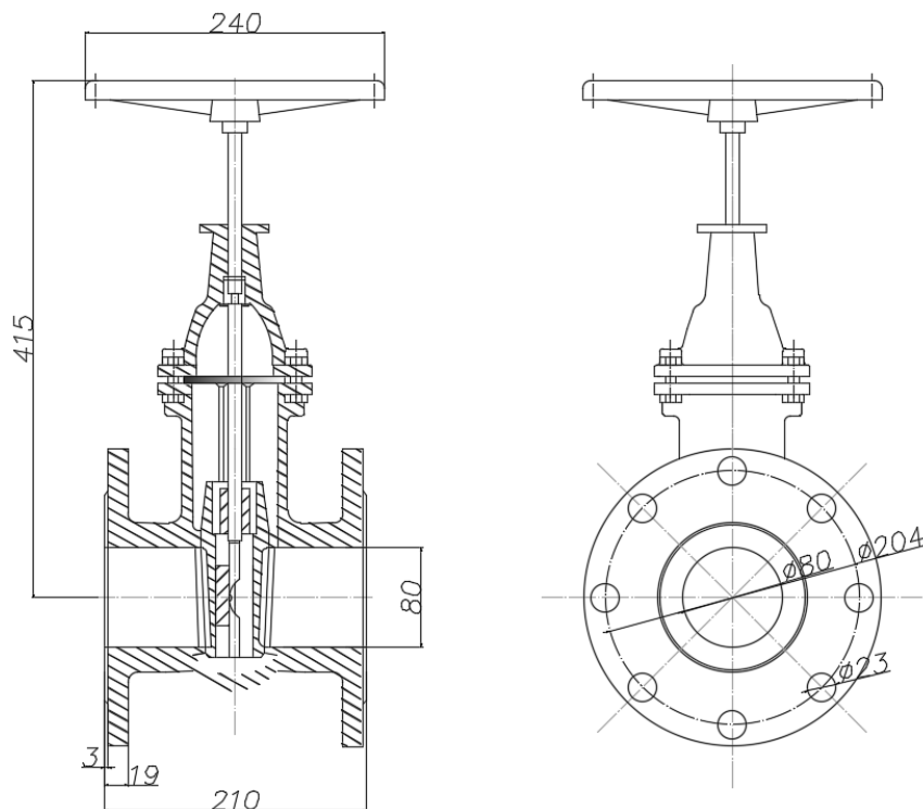
Рис. 13. Клинетная задвижка
